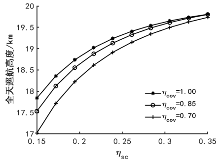
图7 全天巡航高度与 \eta_{sc} 和 \eta_{cov} 的关系 Fig. 7 Relationship between cruising altitude and \eta_{sc} and \eta_{cov}
